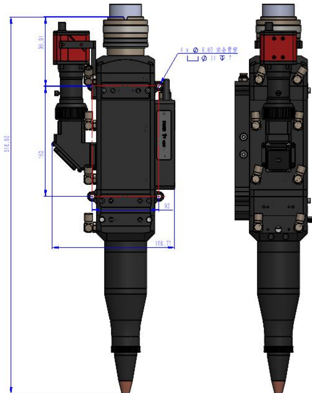
焊接头主要尺寸示意图（准直100/聚焦F300）
