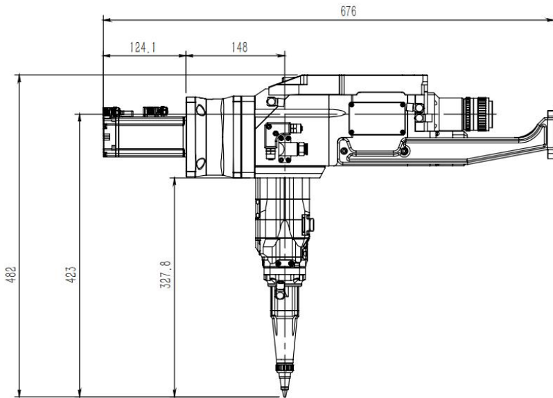
② F300焦安装示意图
